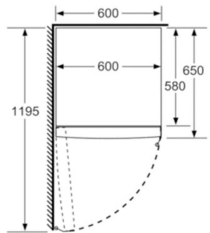
Dimensiones en mm
