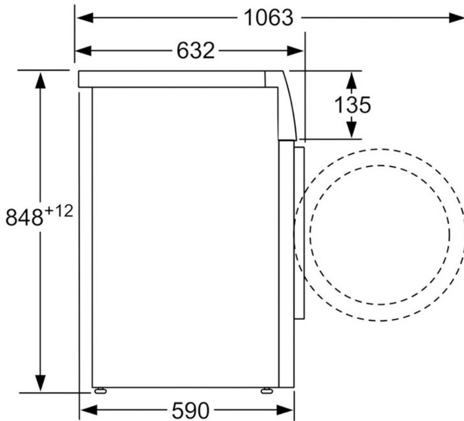
Dimensiones en mm
