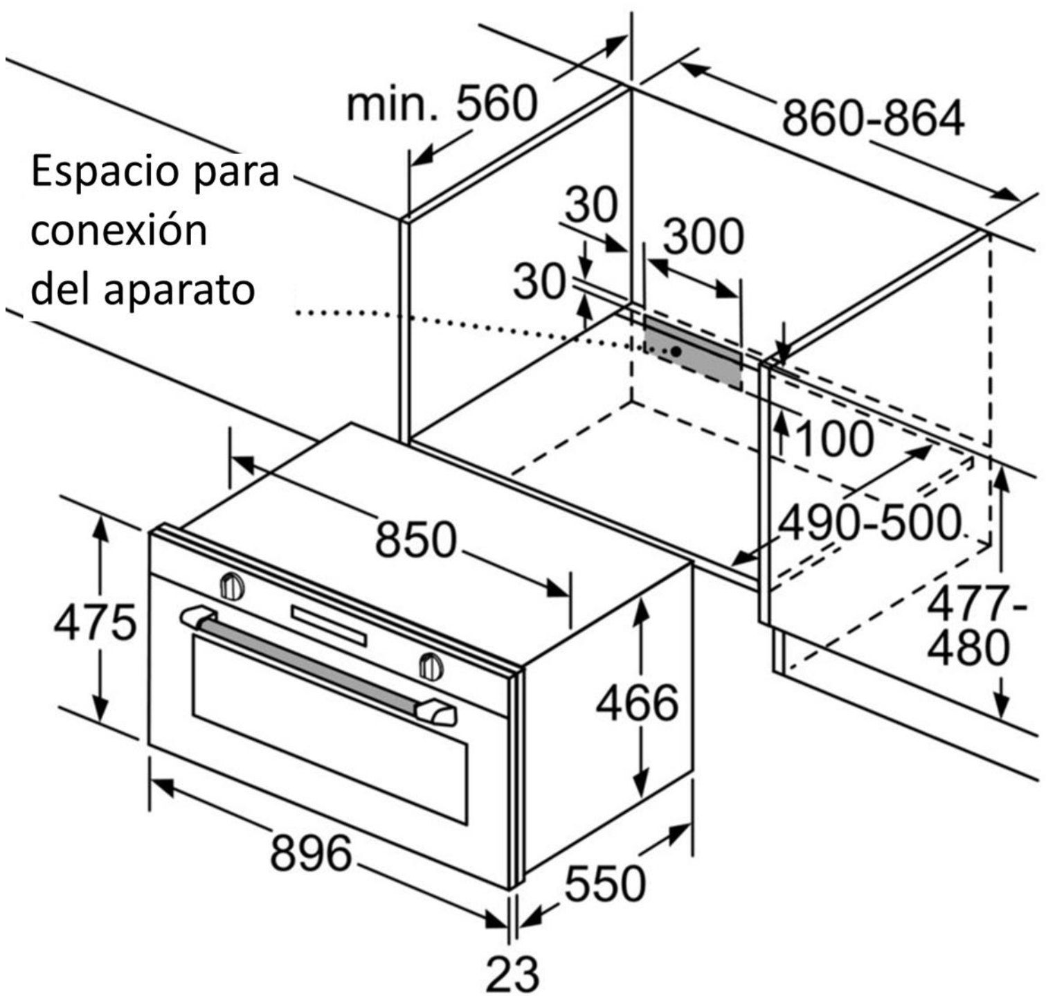
Dimensiones en mm
