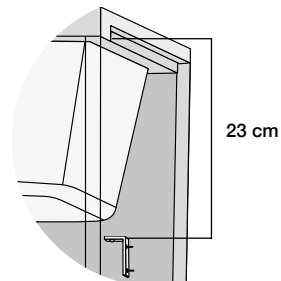
Posición de escuadras para encimeras recrecidas, a 4 cm del postizo.
