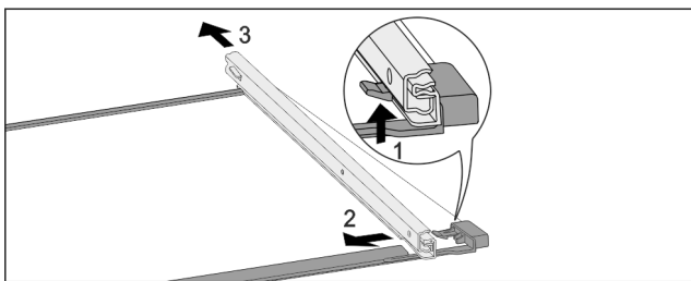
Fig. 150 Placa de vidrio con guías
