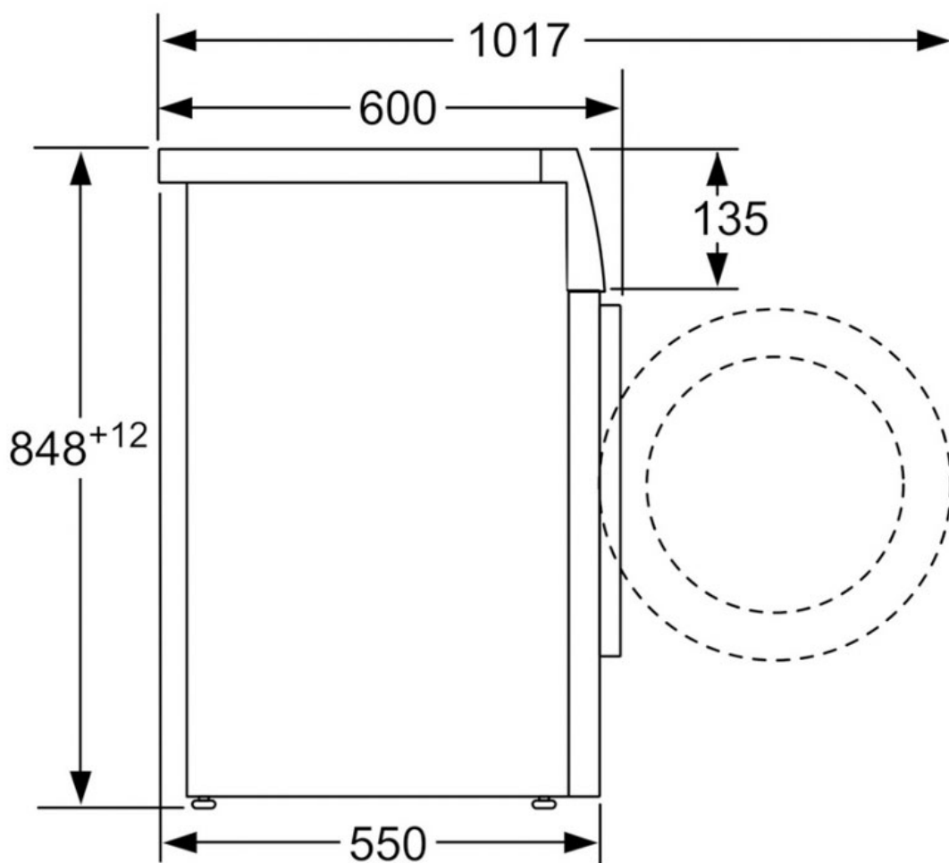
Dimensiones en mm
