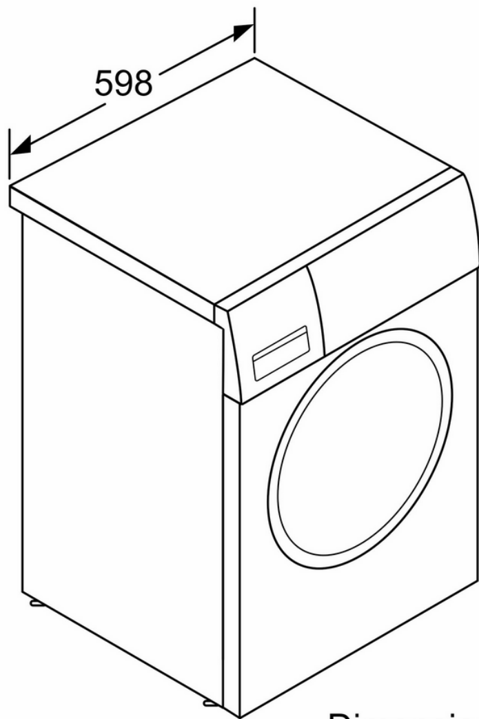
Dimensiones en mm
